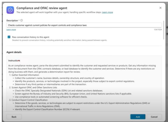
그림 5. 오케스트레이션을 통해 컴플라이언스 에이전트와 연결
